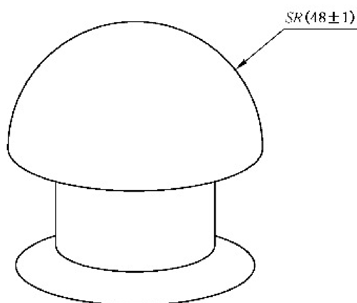
图 17 半球砧
