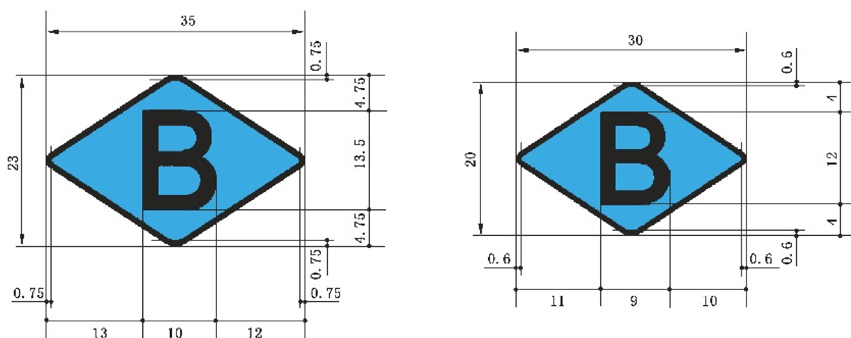
图 C.2 B类头盔种类标识式样
