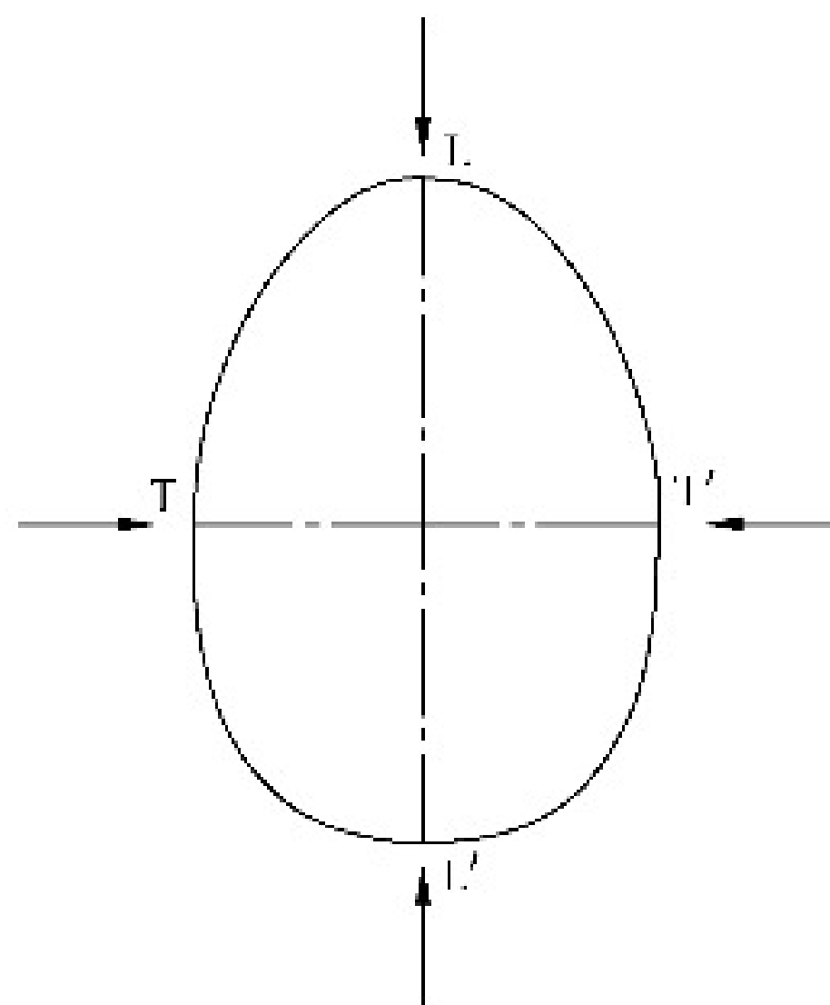
图 12 刚度性能测试
