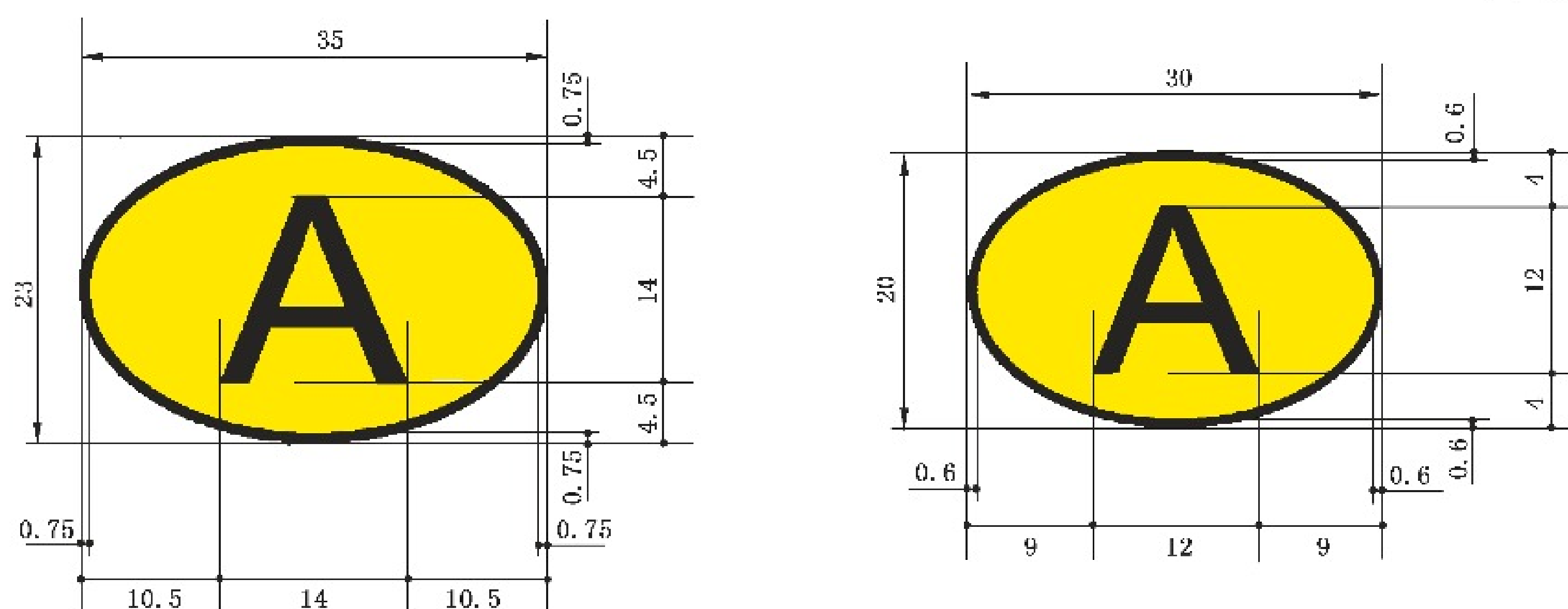
图 C.1 A类头盔种类标识式样
