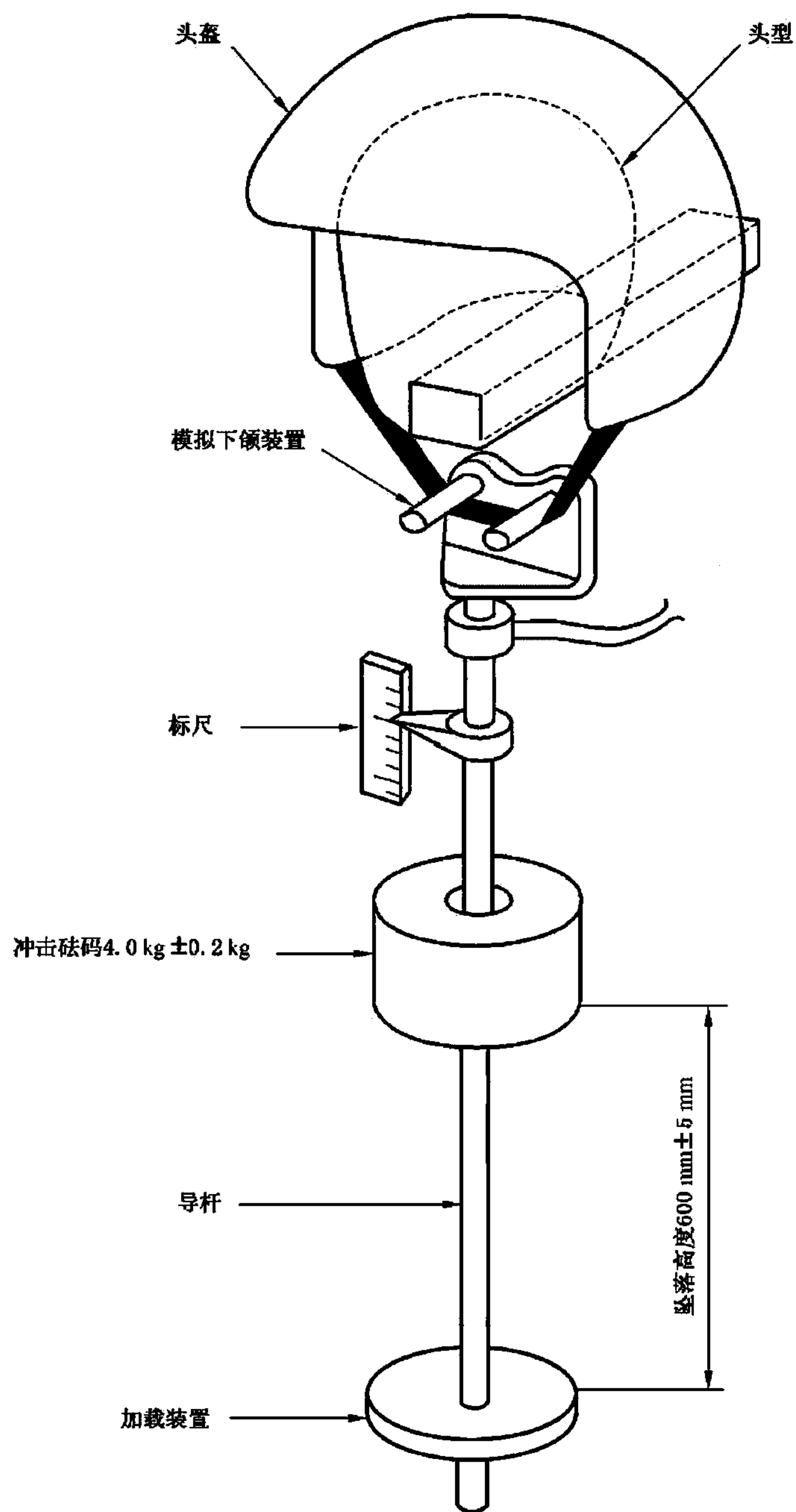
图 7 佩戴装置强度试验台
