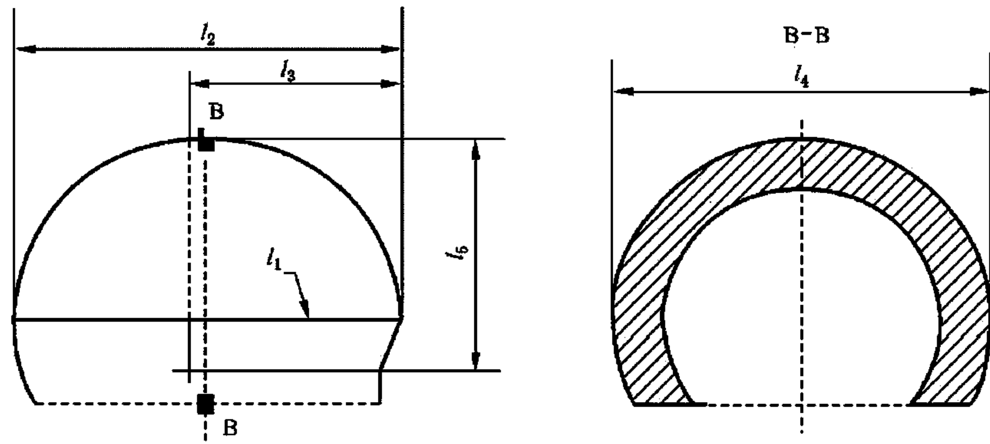
图 9 头型
