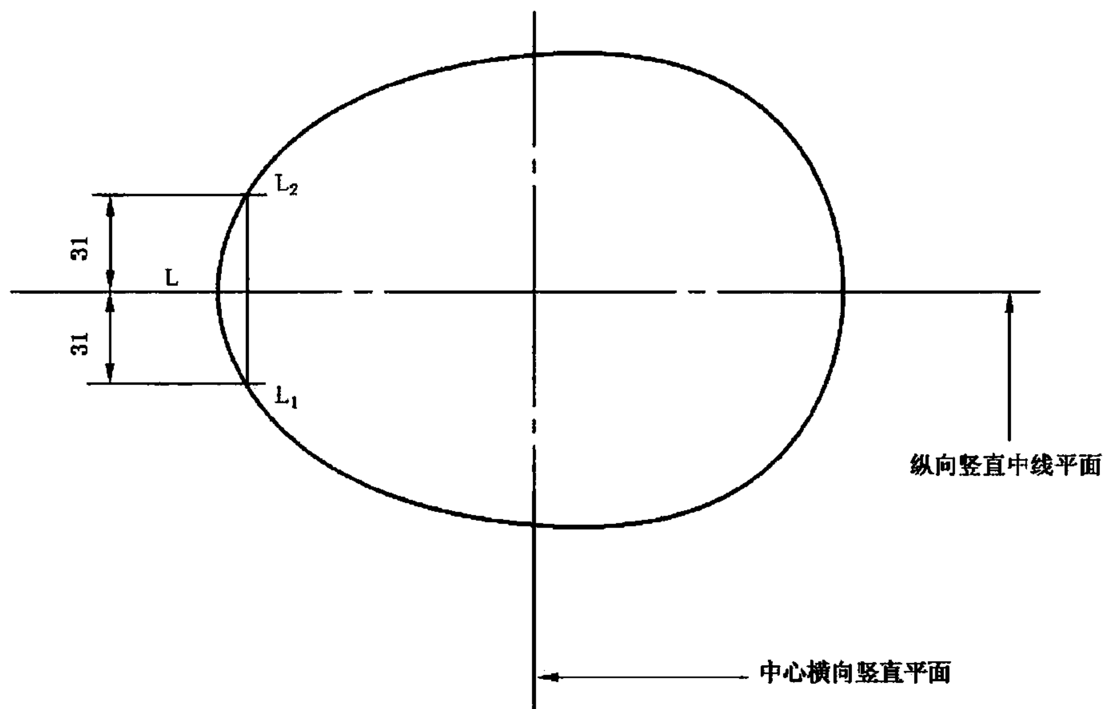
b) 头型剖面俯视图
