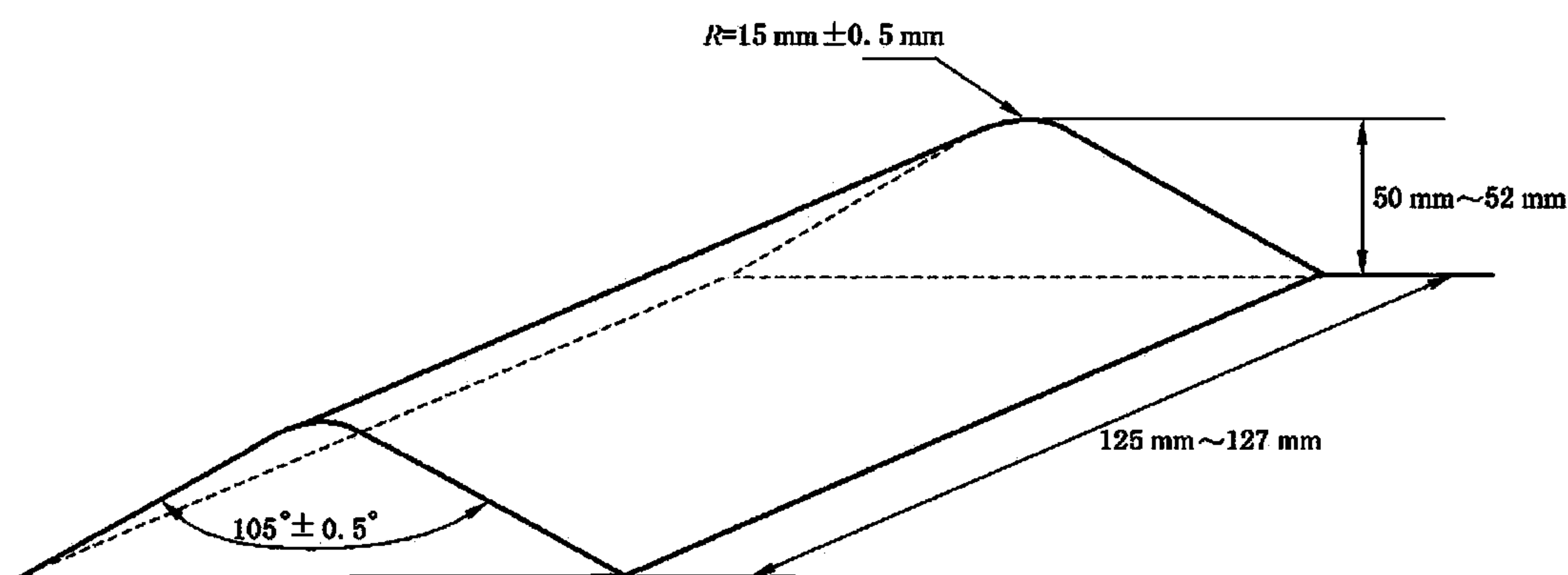
图 11 路缘石砧
