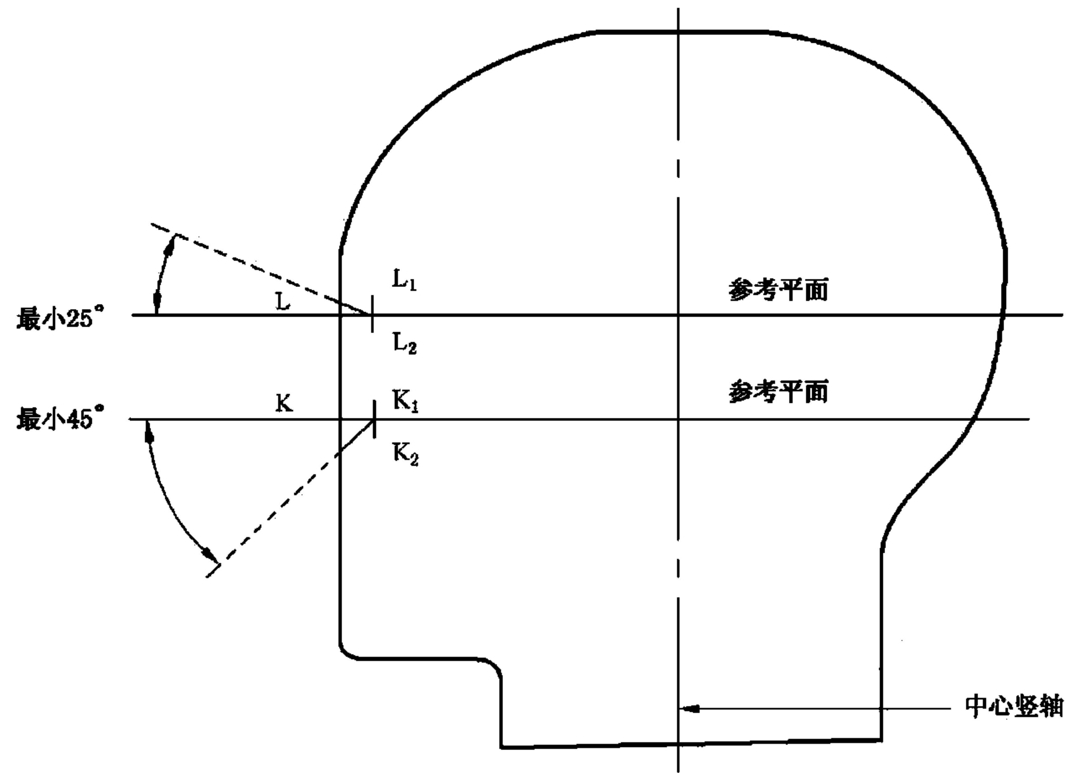
a) 纵向垂直平面中的头型剖面图
