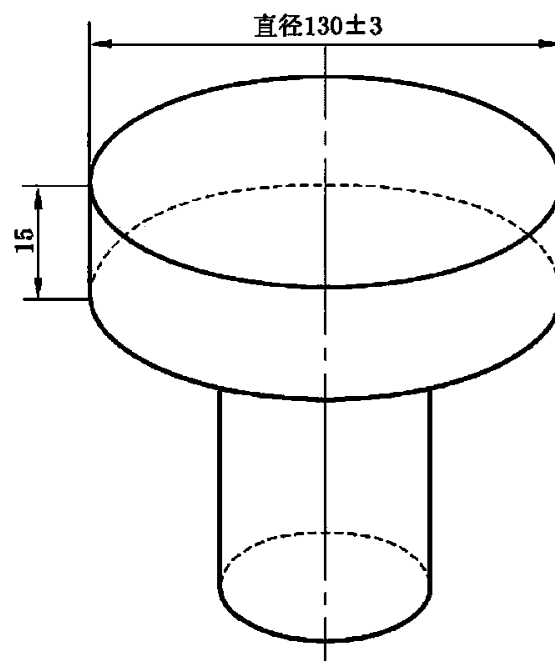
图 10 平砧
