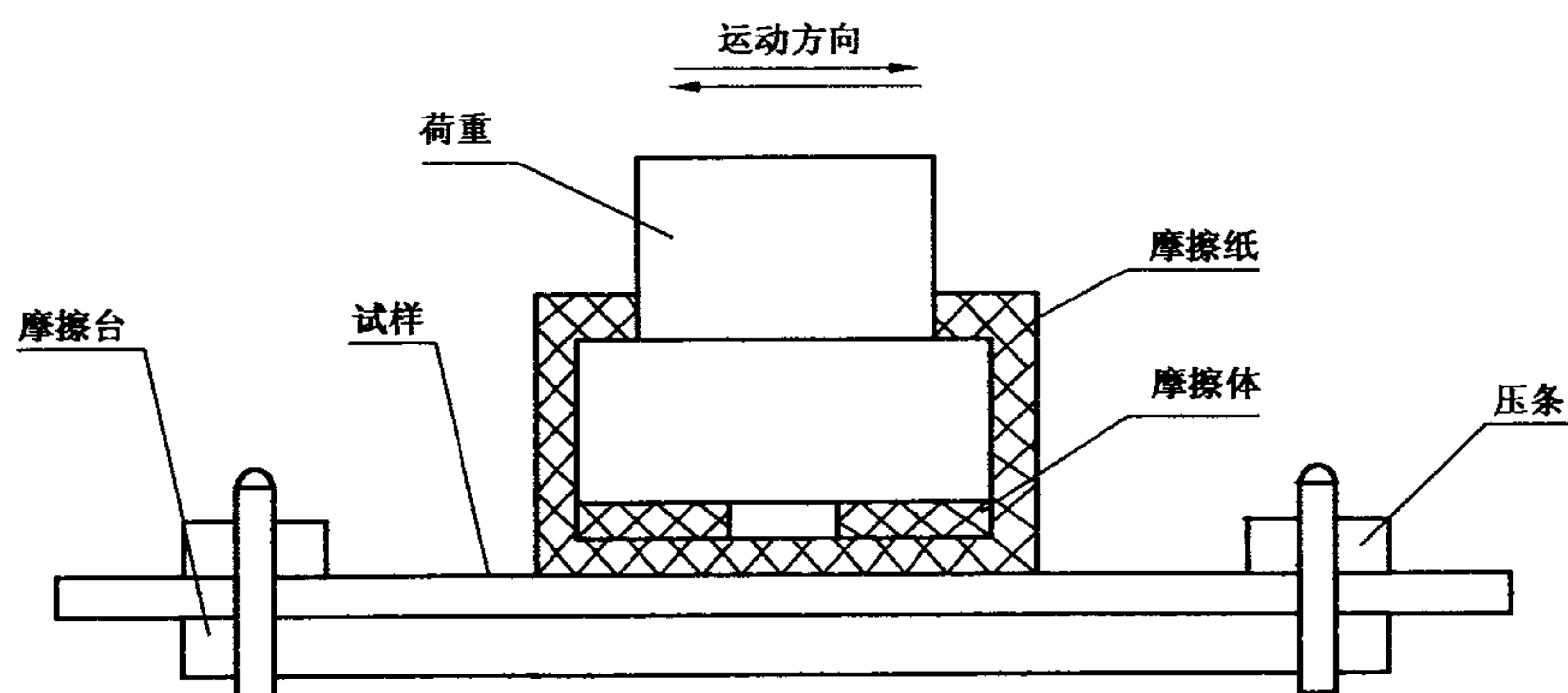
图 1 摩擦检验机
