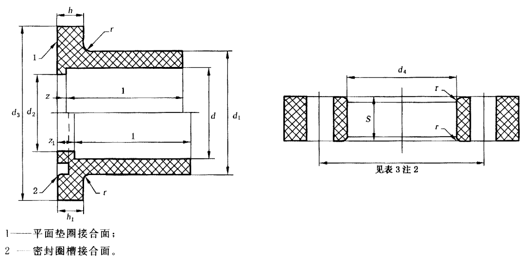
图 2 活套法兰变接头
